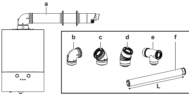
a Wandanschluss-Kit 60/100
