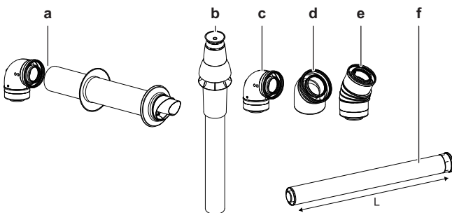
a 60/100-auf-80/125-Adapter
